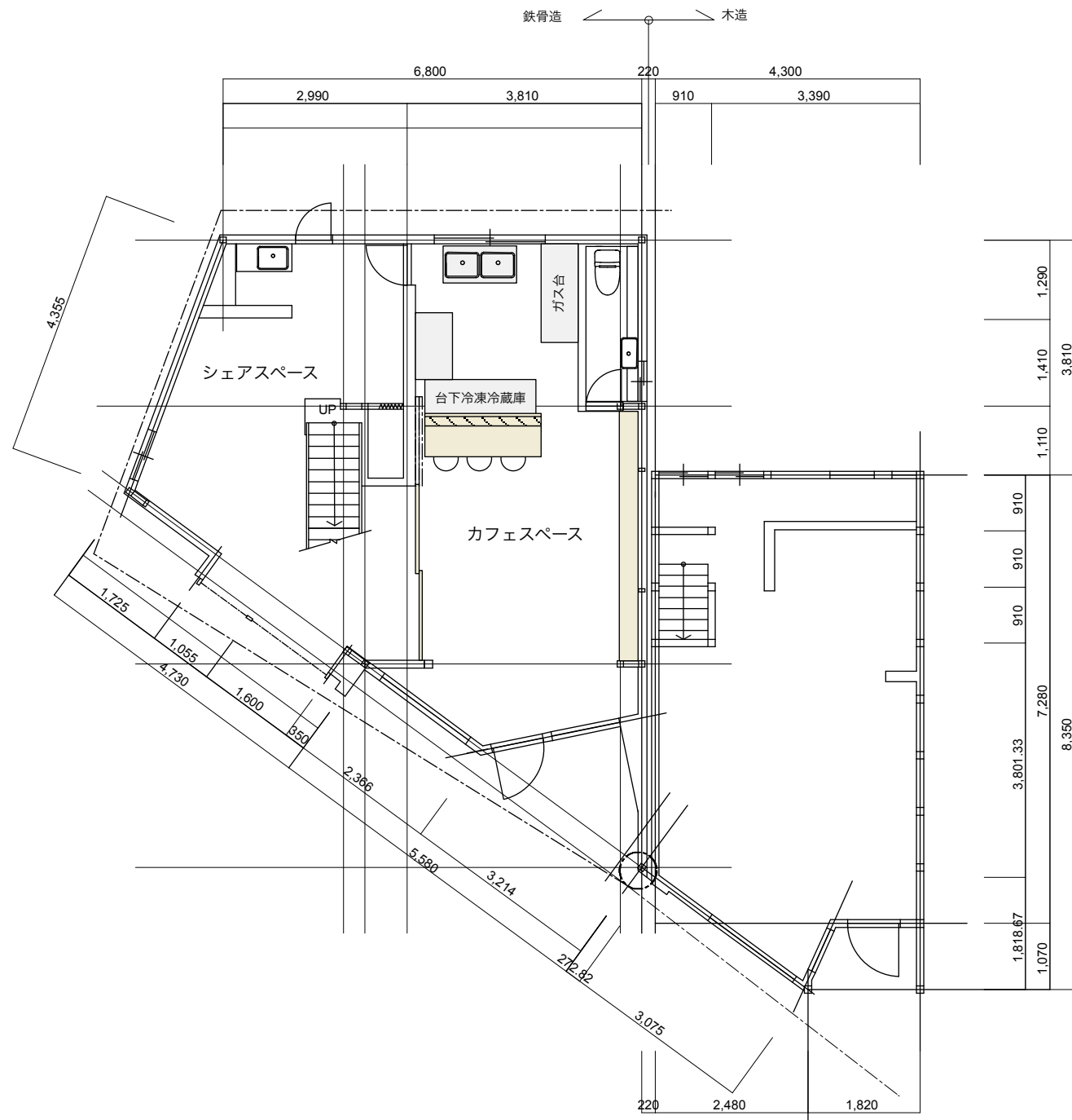
1階平面図
