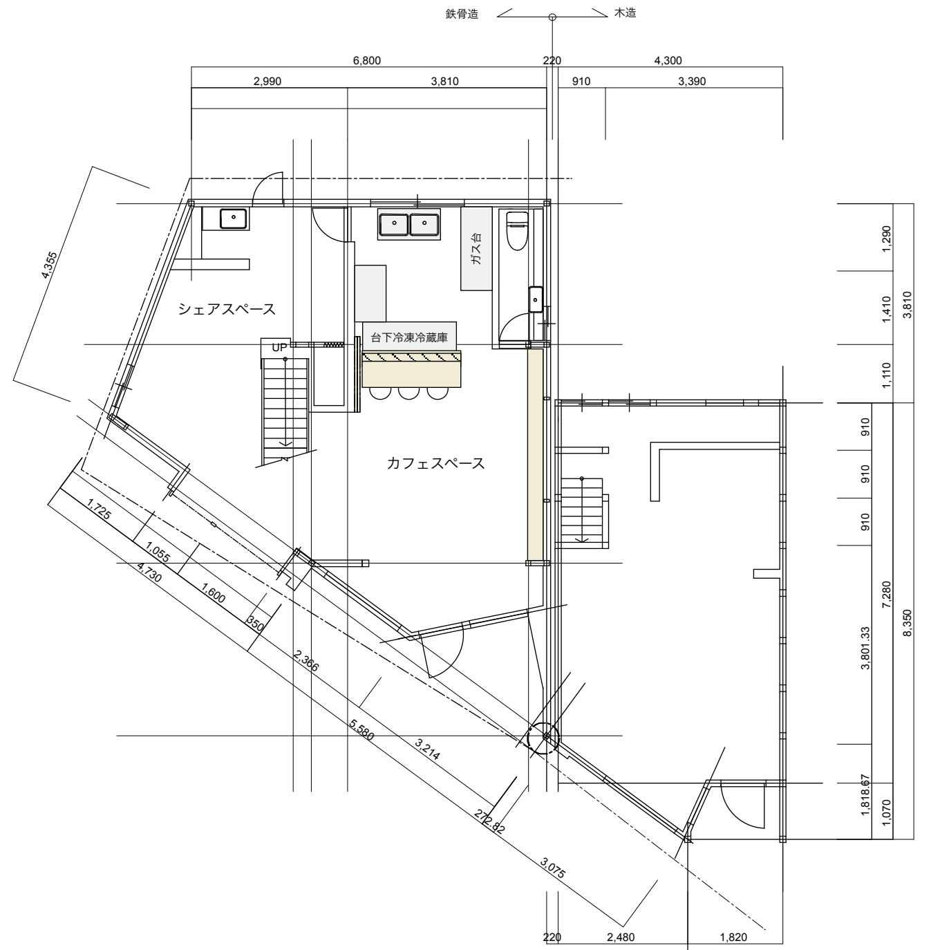
1階平面図
